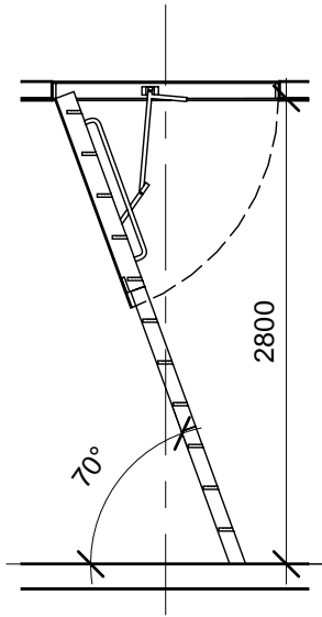
RN28 Section 1 : 50
