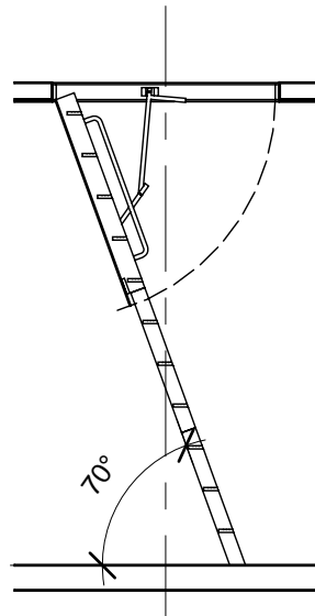
R27 Section 1 : 50
