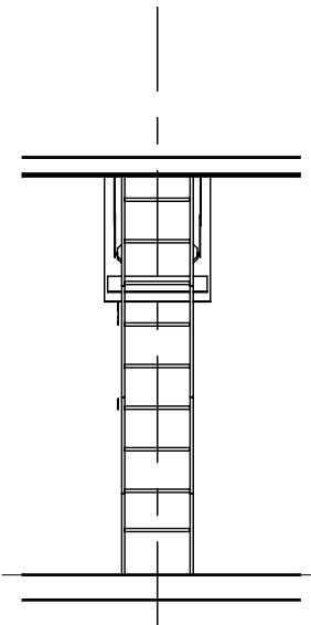
Q24 Front 1 : 50
