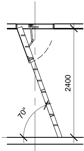
Q24 Section 1 : 50
