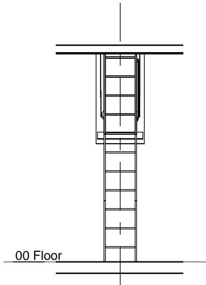
D27 Front 1 : 50
