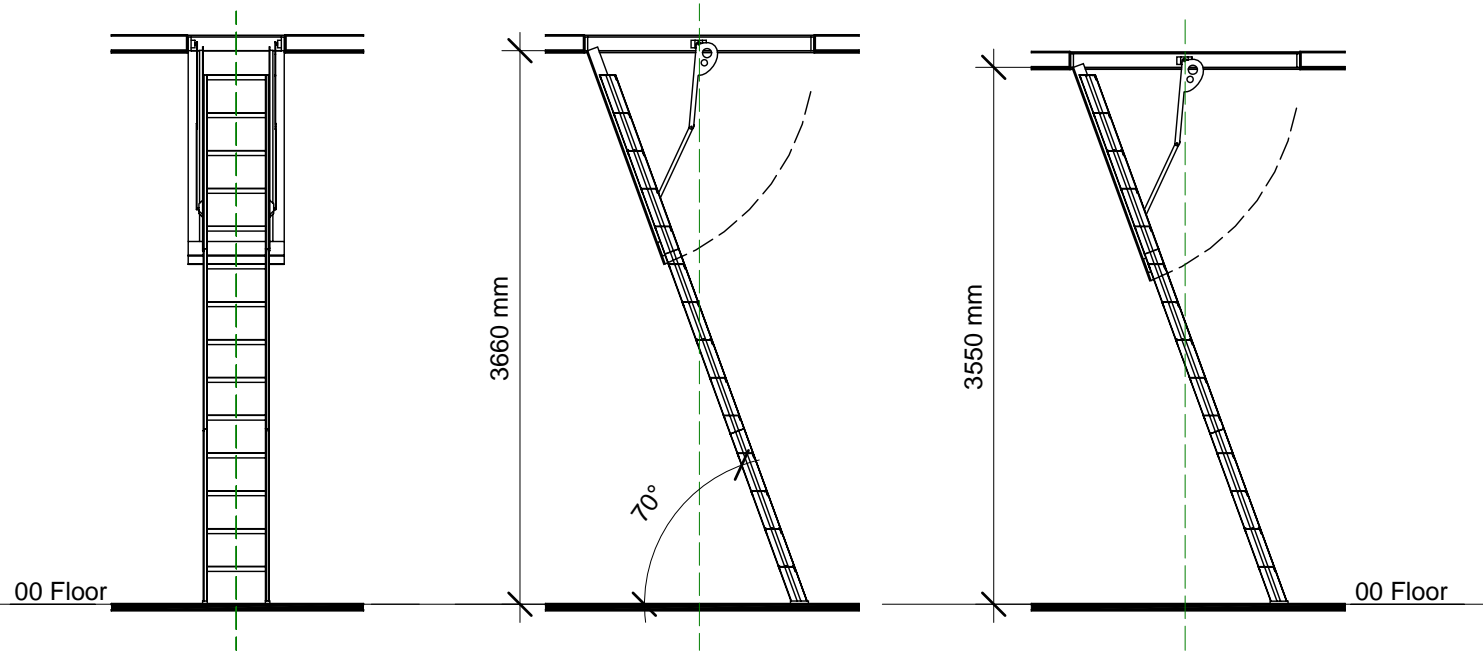
A36 Front 1 : 50
